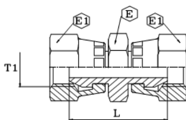
Adaptor metric DKOL - METD filet interior, cu olandeză con 24 de grade
