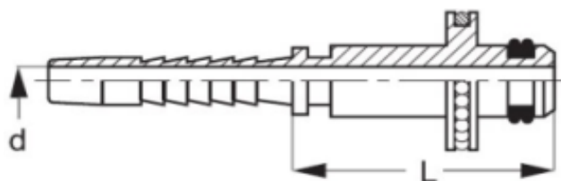
Armătură TIPOGUN cu rulment -garnitură O-ring -inel teflon pentru ștuț 11 mm
