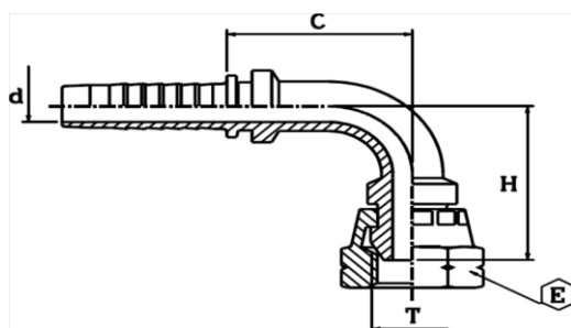
Armătură MULTISEAL, DKL90 DIN 3868 con 24/60 de grade
