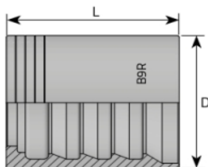
Bucșă 4SP/4SH - BPR pentru furtunuri tip EN 856: 4SP-4SH cu decojire
