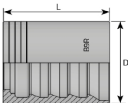
Bucșă 4SP - BP2 pentru furtunuri tip EN 853: 4SP cu decojire
