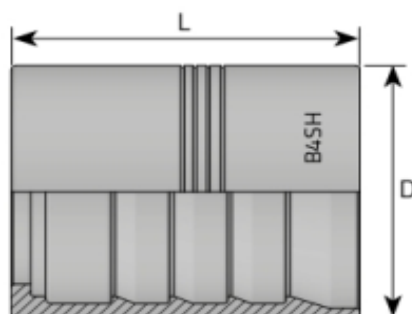
Bucșă 4SH - BPR pentru furtunuri tip EN 856: 4SH cu decojire
